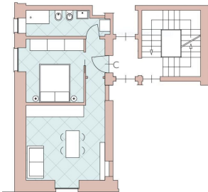
PIANTA PIANO SECONDO - ARENZANO, VIA DELLE OLIVETTE 23
